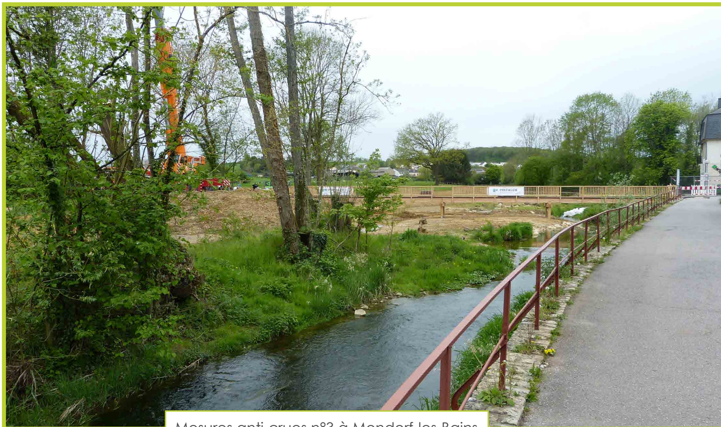
Mesures anti-crues n°3 à Mondorf-les-Bains
